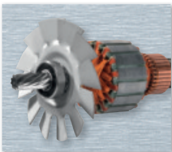
Metalni ventilator u 66 mm cirkularnoj testeri.
